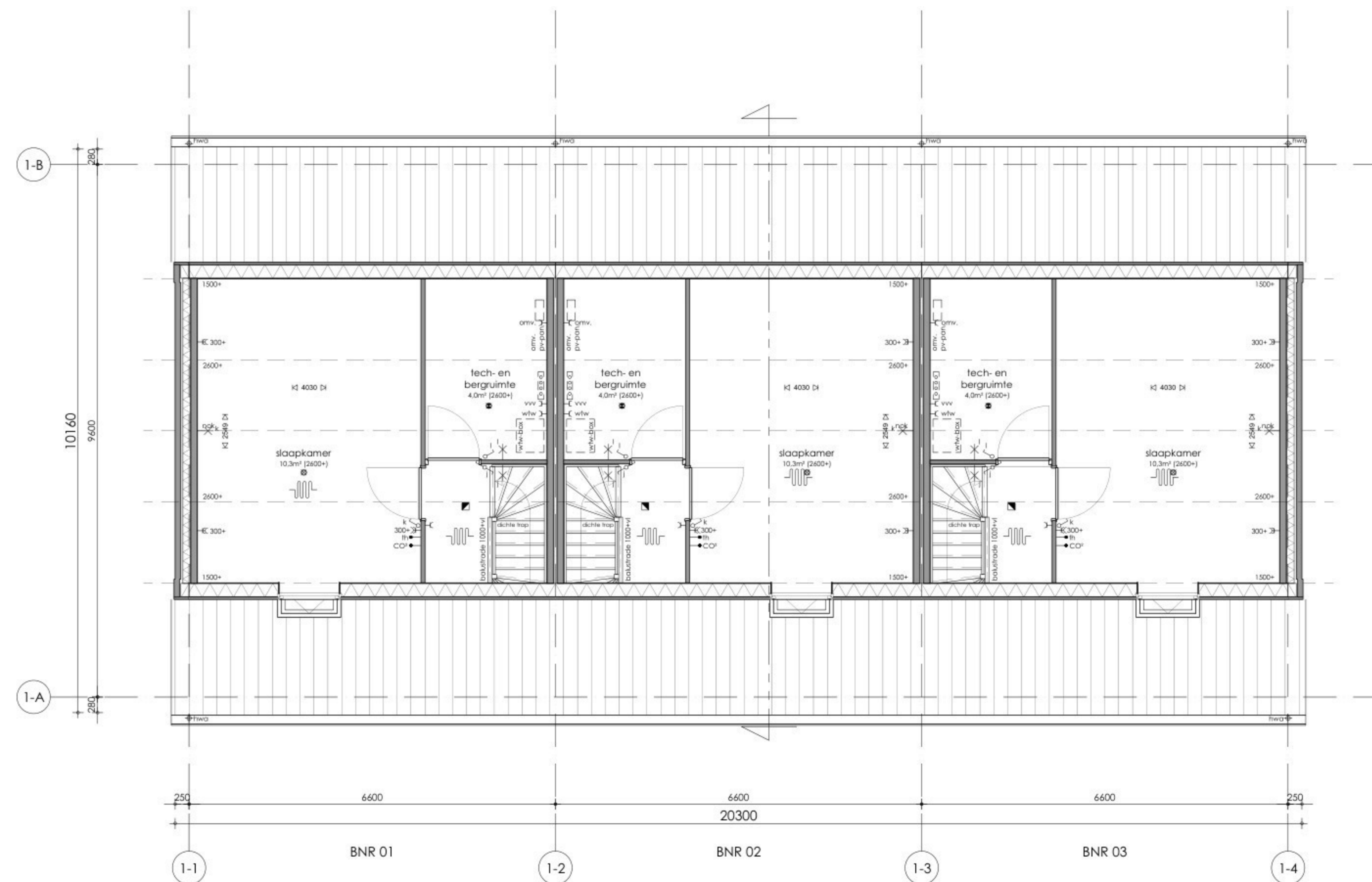
1E VERDIEPING
