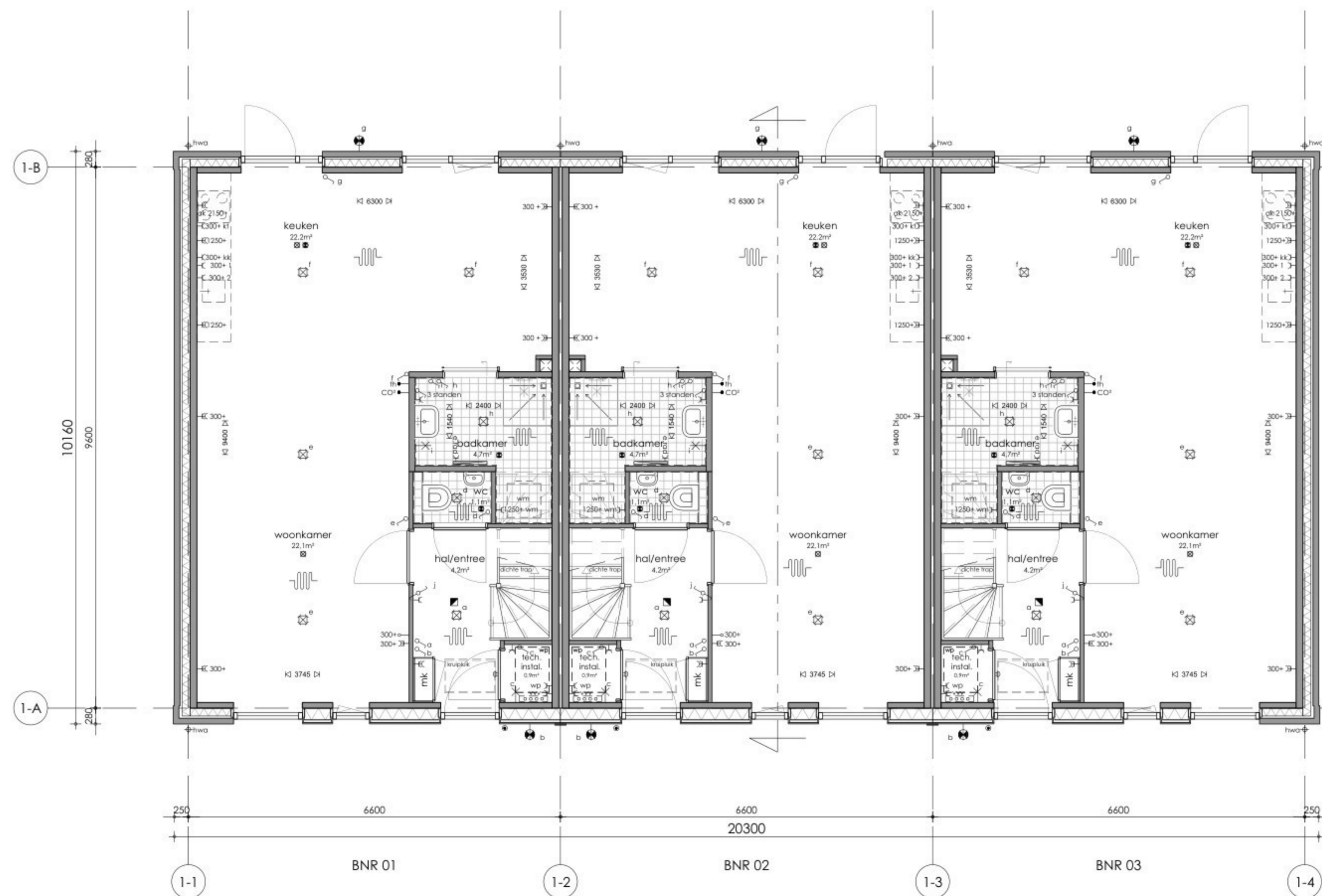
BEGANE GROND
