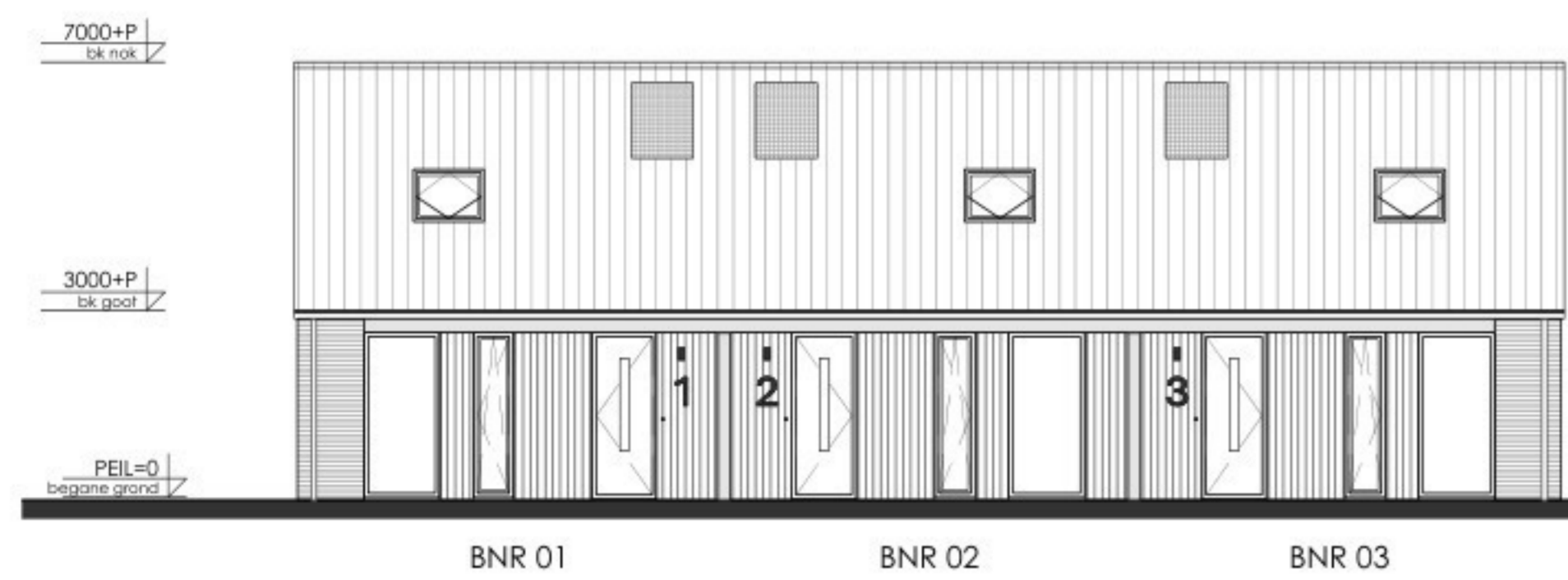
VOORGEVEL | ZUIDOOST
