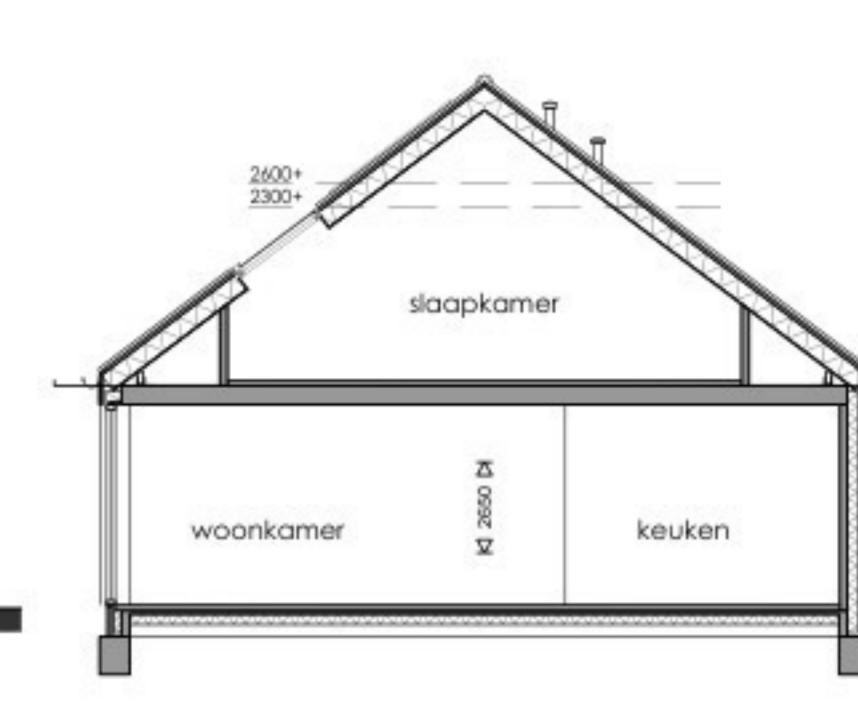
DOORSNEDE
