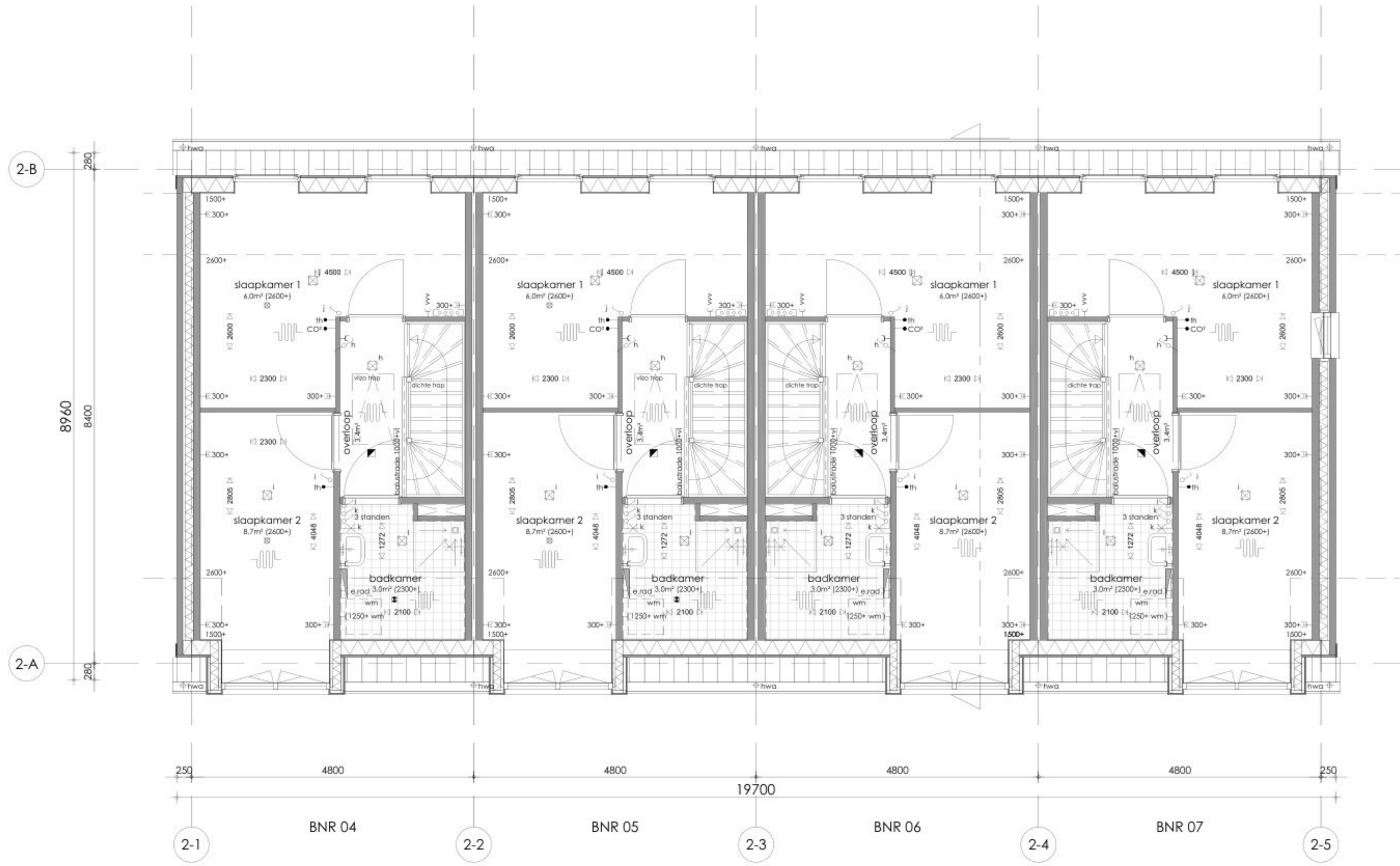
1E VERDIEPING
